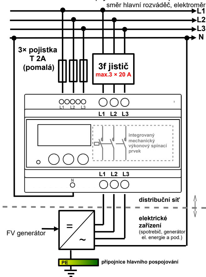
Obr. 1: Schéma zapojení zařízení ochrany
